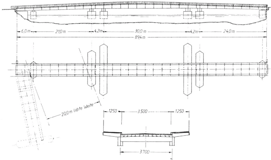
2 Schwimmbrücke über die Ruhr in Dahlhausen, mit ausschwimmbarem Teil, Aufriss, Grundriss, Querschnitt.
